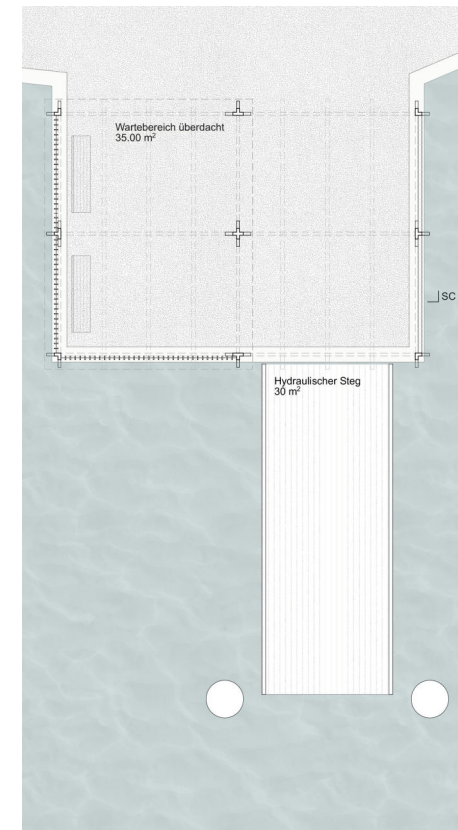
Grundriss Schiffflände
