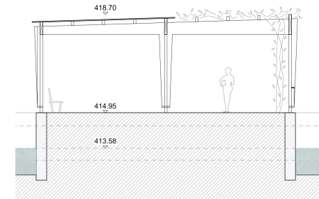
Schnitt Schiffflände
